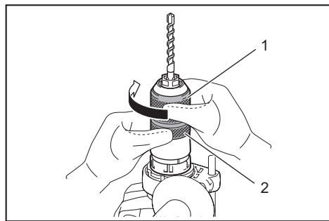
► 1. Mandril 2. Anillo
