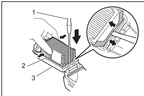
► 1. Destornillador de punta plana 2. Caja del filtro 3. Cubierta de la caja para polvo
